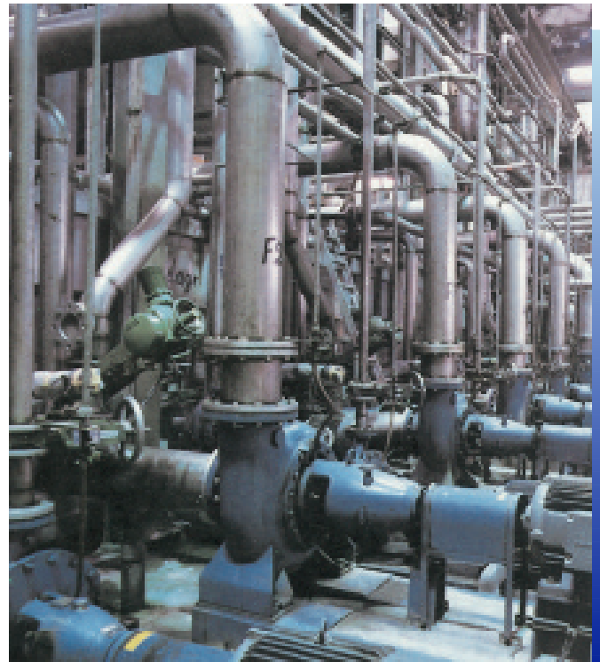
Verrohrung im konstanten Teil einer Kartonmaschine/ Piping system in paper plant
